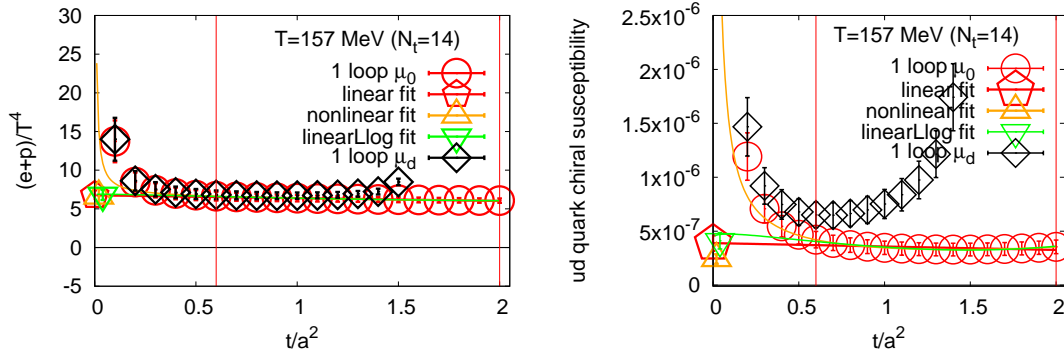
図 4: グラジエントフローに基づく SFtX 法による有限温度 (2+1)-flavor QCD の研究: 現実のクォーク質量におけるくりこみスケール依存性。左図: エントロピー密度 \epsilon + p 。右図: ud クォークのカイラル感受率の非連結部分。 T = 157 MeV での結果。横軸は無次元の flow-time t/a^2 で、物理的結果は t \rightarrow 0 外挿によって得られる。(論文 12)
