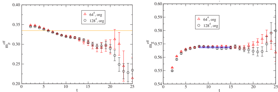
図 1: 格子サイズ 128^4 と 64^4 における \rho メソン局所有効質量(左)と三バリオン局所有効質量(右)。
