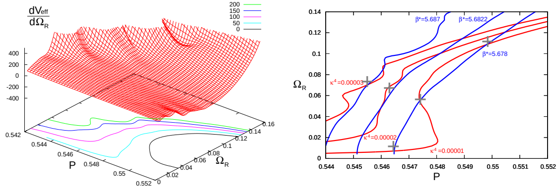
図 4: ヒストグラム法によるクォークが重い領域の QCD における有限温度相構造の研究 (論文 7)。(左) プラケット (ゲージ場のエネルギー) とポリアコフループ (重いクォークのエネルギー) に関する有効ポテンシャルのポリアコフループに関する微分と、ポリアコフループ方向の傾き一定の線。(右) 前述の有効ポテンシャルにおけるプラケット方向とポリアコフループ方向の傾き一定の線。詳細は本文参照。
