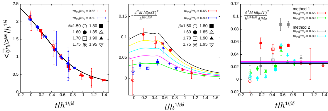
図 3: 2 フレーバー QCD の有限温度・有限密度カイラル相転移近傍のスケーリング（論文 6）：(左図) カイラル凝集の O(4) スケーリング。 \mu_q/T < 1 の全データが示されている。誤差の大きなデータは \mu_q/T \sim 1 のもの。曲線は O(4) スピン模型のスケーリング関数。(中央) カイラル凝集の \mu_q/T に関する 2 次微分係数。method 1 の結果。 \mu_q/T < 1 (右図) 係数 c 。
