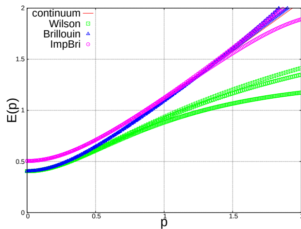
図 9: 自由場上で分散関係。 m_q a = 0.5 。
