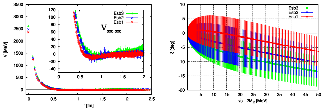
図 7: ^3S_1 チャンネルにおける \Xi\Xi 間のポテンシャルと散乱位相差。
