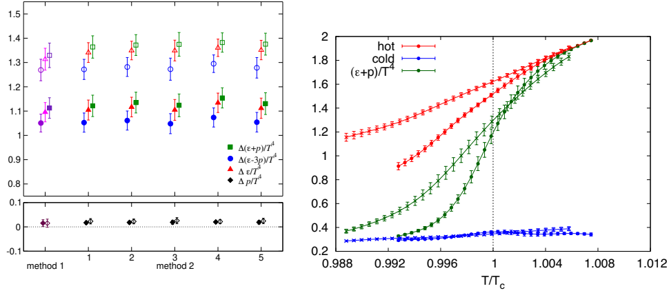
図 3: クエンチ近似 QCD の潜熱と圧力ギャップに関して a \rightarrow 0 と t \rightarrow 0 の2重外挿を行った最終結果。左図: t \rightarrow 0 を先に実行する”method 1”と a \rightarrow 0 を先に実行する ”method 2” の結果の比較 (method 2 では、さらに t \rightarrow 0 外挿のフィット・レンジをいくつか比較)。filled symbols はアスペクト比 N_s/N_t = 8 、open symbols は N_s/N_t = 6 に相当する空間体積での結果。右図: N_t = 8 格子におけるエントロピー密度のヒステリシス。空間体積が小さい N_s/N_t = 6 格子 (細いシンボル) と空間体積が大きい N_s/N_t = 8 格子 (太いシンボル) の比較 (論文 [6])。
