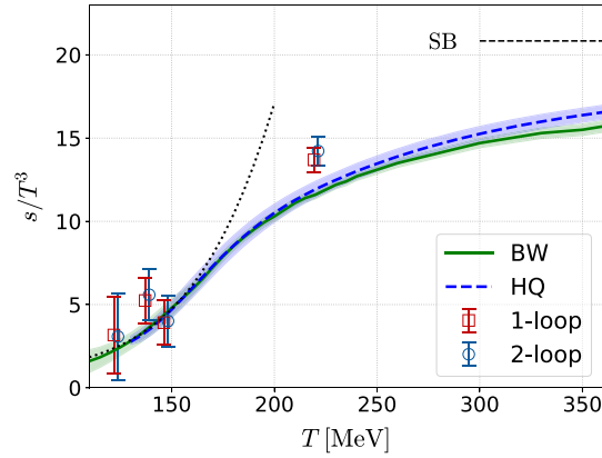
図 2: SFtX 法を用いた物理点 N_f = 2 + 1 QCD の有限温度シミュレーション。低温領域 ( T = 122, 137 MeV) の統計を改善したエントロピー密度。Budapest-Wuppertal Collaboration と HotQCD Collaboration による、先行結果（通常の方法を採用し、スタガード型クォークを用いている）との比較（学会発表 [27] で示した中間結果）。この後に統計はさらに改善されている。
