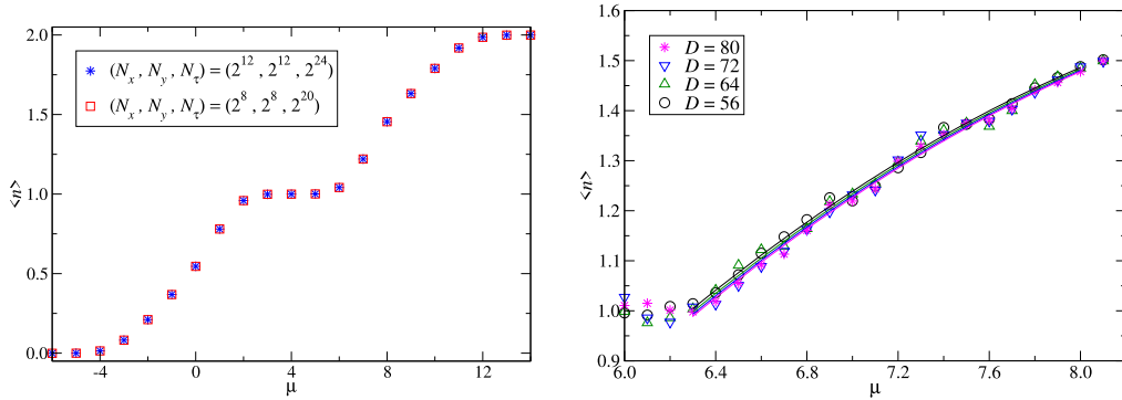
図 8: (左) U = 8 における電子密度 \langle n \rangle を化学ポテンシャル \mu の関数としてプロットしたもの。 D_{\text{cut}} = 80 で格子サイズは (N_\sigma = N_{x/y}, N_\tau) = (2^{12}, 2^{24}) (青) と (2^8, 2^{20}) (赤) の2種類。(右) 6.0 \leq \mu \leq 8.0 の領域において左図よりも \mu の解像度を上げて電子密度 \langle n \rangle を計算した結果。曲線は \mu と D_{\text{cut}} (= D) に関する global fit の結果を表す(論文[13])。
